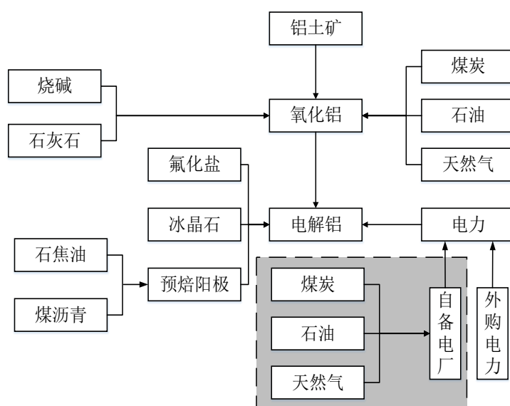
图3 电解铝生产企业碳排放源结构
